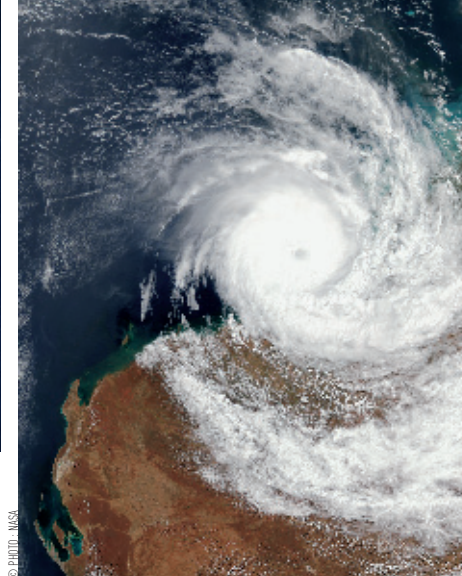
Cyclone tropical de catégorie 4 sur la côte australienne en mars 2004.
