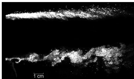
L'image du haut montre un écoulement fluide supersonique relativement régulier. Dans l'image du bas, l'action d'un petit jet de fluide injecté latéralement a eu pour résultat le développement d'instabilités dans l'écoulement. Une telle manipulation illustre l'idée que l'on peut agir sur un écoulement à l'aide de petits dispositifs, notamment en vue de le contrôler (Cliché Erwan Collin-LEA/CEAT-Université de Poitiers).
